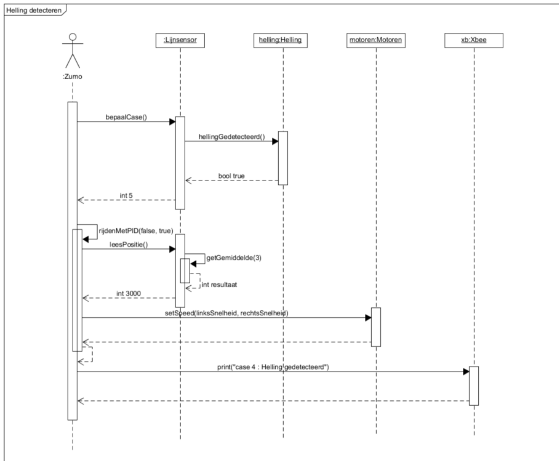
Figuur 3: Sequentiediagram hellingdetectie
